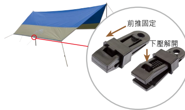
DJ-5061 4716804050610 天幕夾/帳篷夾(5入) 尺寸：約長8.5×寬3.2×高2.1cm 咬合鋸齒面積：2.8cm 孔洞直徑：1cm 重量：約22g/單個；約110g/5入 材質：ABS · 用於無綁繩扣、無銅卸布幕 · 輕鬆夾上·即可固定 · 適用帆布、天幕布水線、帳棚外帳
